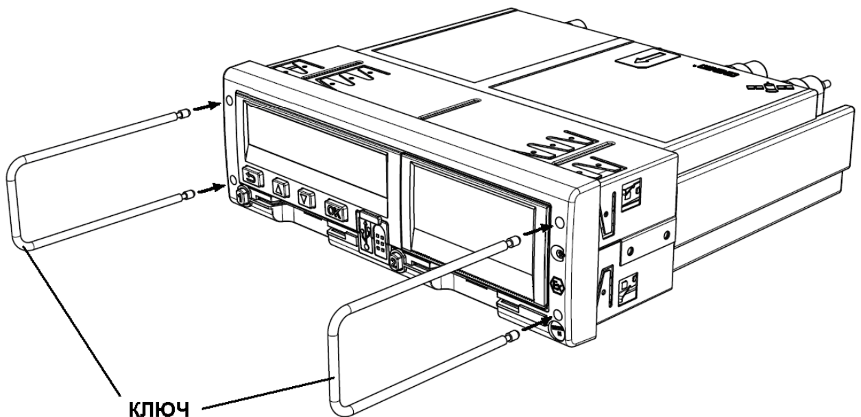
Рисунок 3 – Извлечение тахографа
