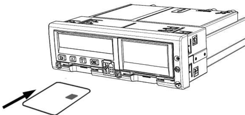
Рисунок 4 – Вставка карты предприятия в картоприемник основного водителя «1»
