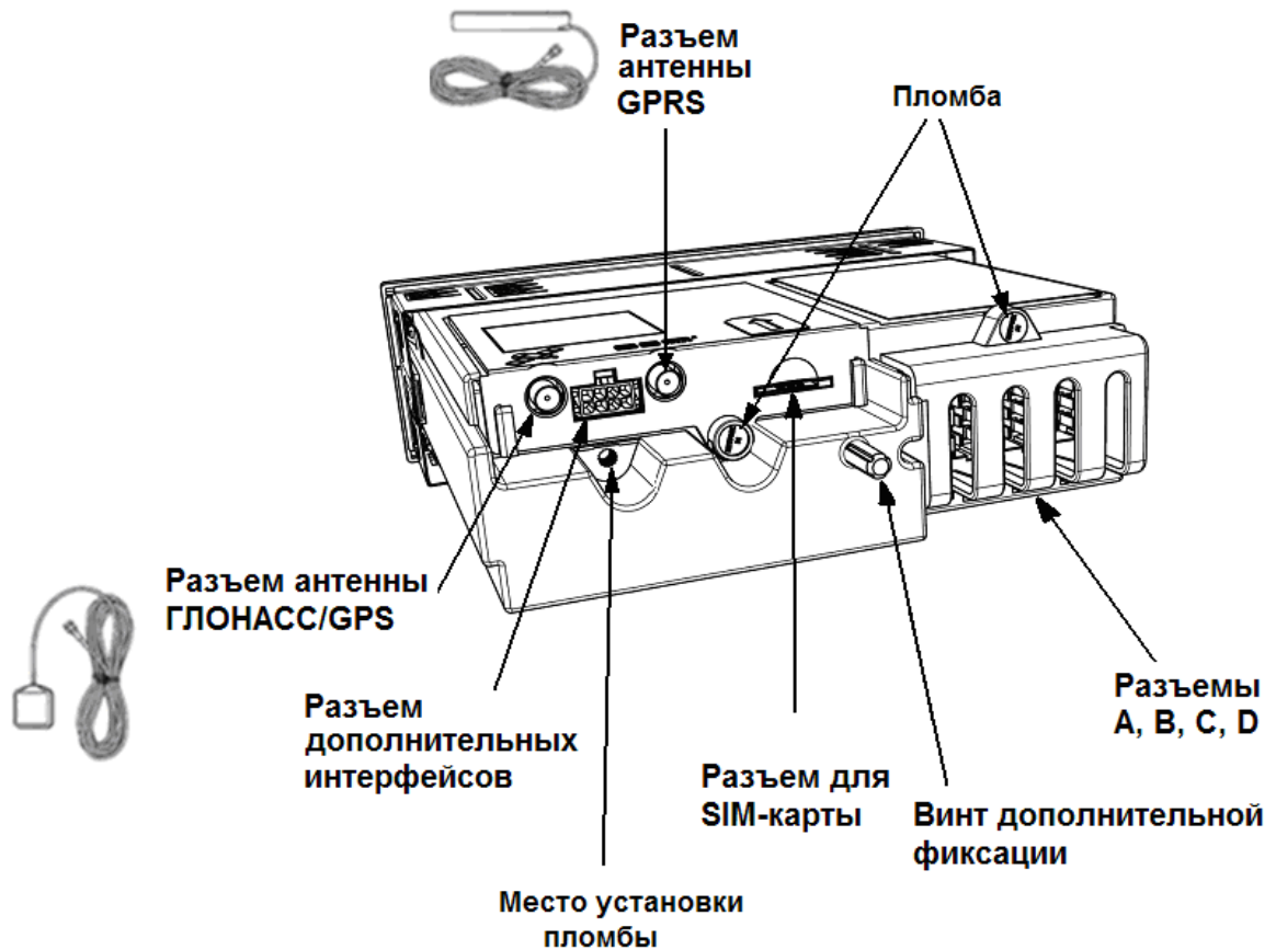
Рисунок 2 – Внешний вид задней панели тахографа
