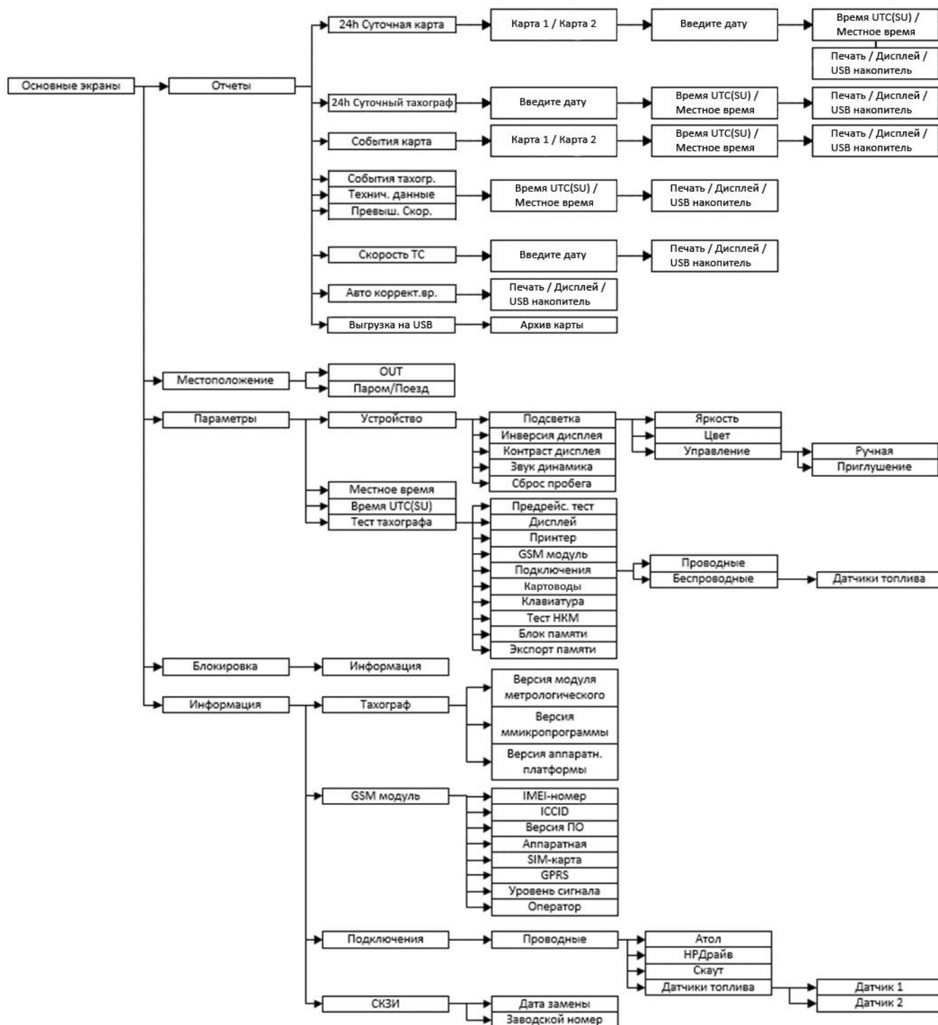
Рисунок 7. Структура меню рабочего режима
