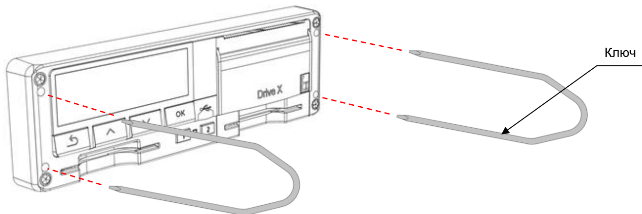
Рисунок 1. Извлечение тахографа
