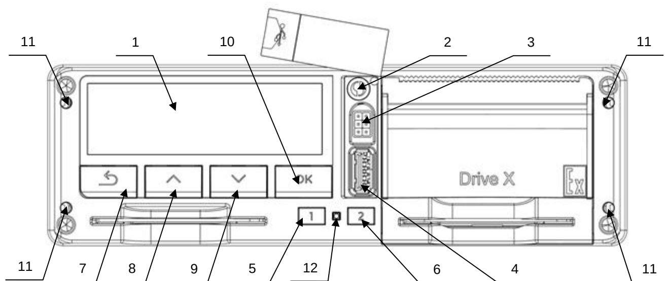
Рисунок 3. Вид спереди
