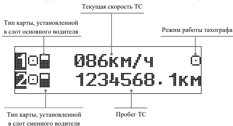
Рисунок 13. Экран скорости и одометра
