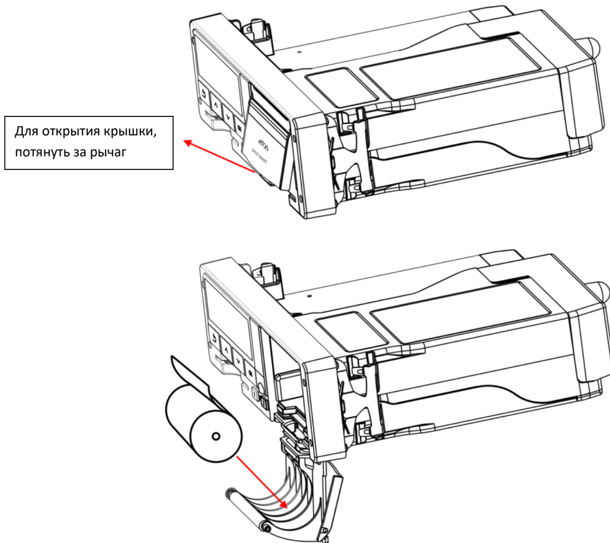
Рисунок 6. Установка бумаги
