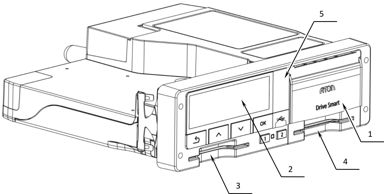
Рисунок 2. Внешний вид тахографа
