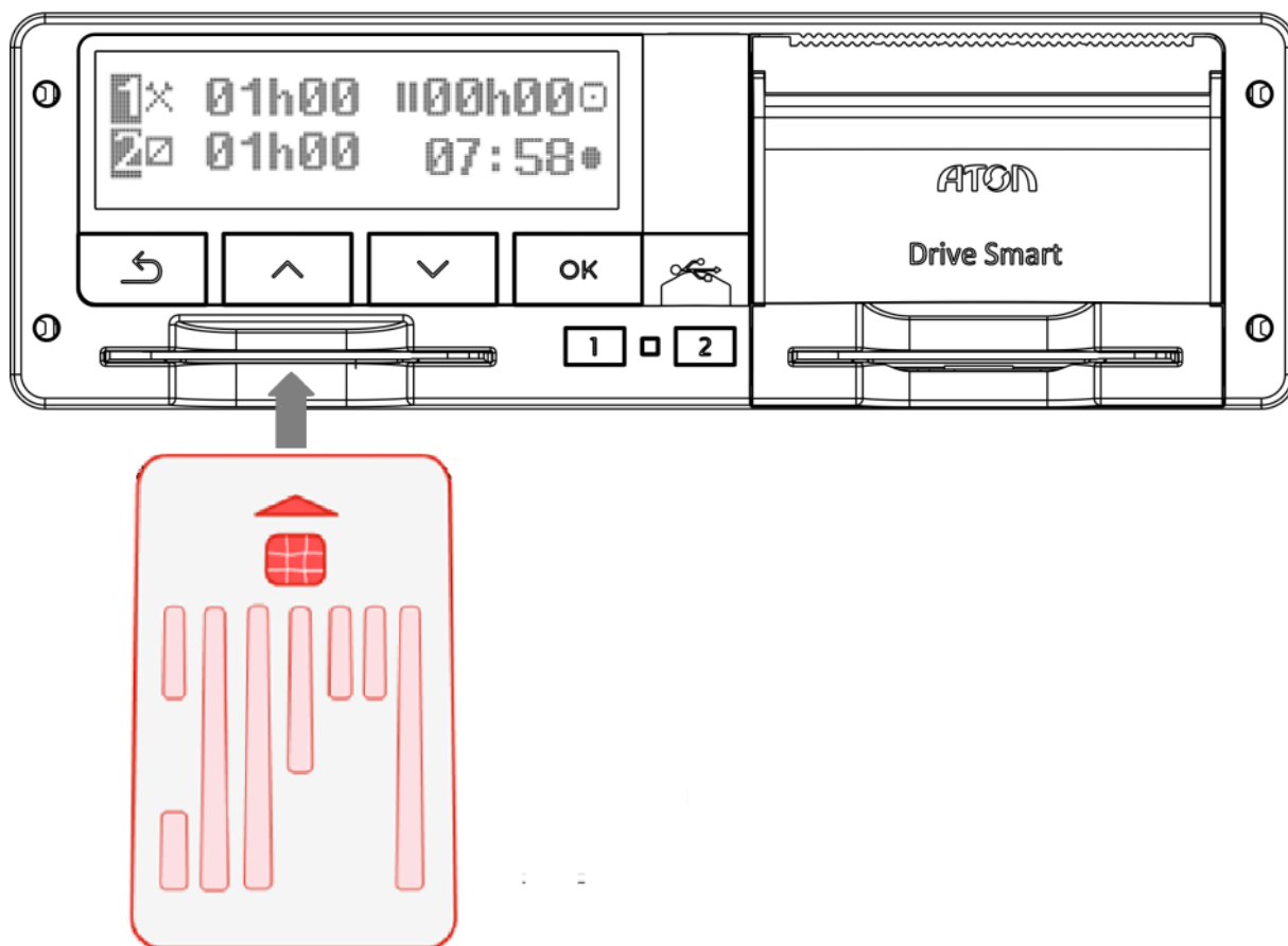
Рисунок 5. Установка карты
