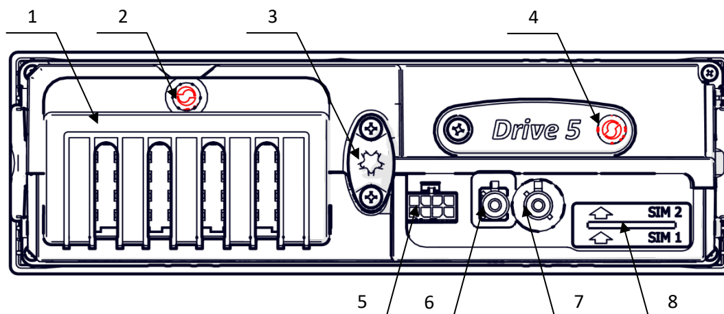
Рисунок 4. Вид сзади
